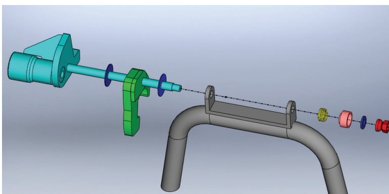
FIGURA 2 ESPLOSO DI MONTAGGIO
